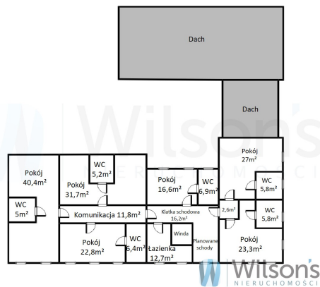
POGLĄDOWY PLAN NIERUCHOMOŚCI- POZIOM +1
